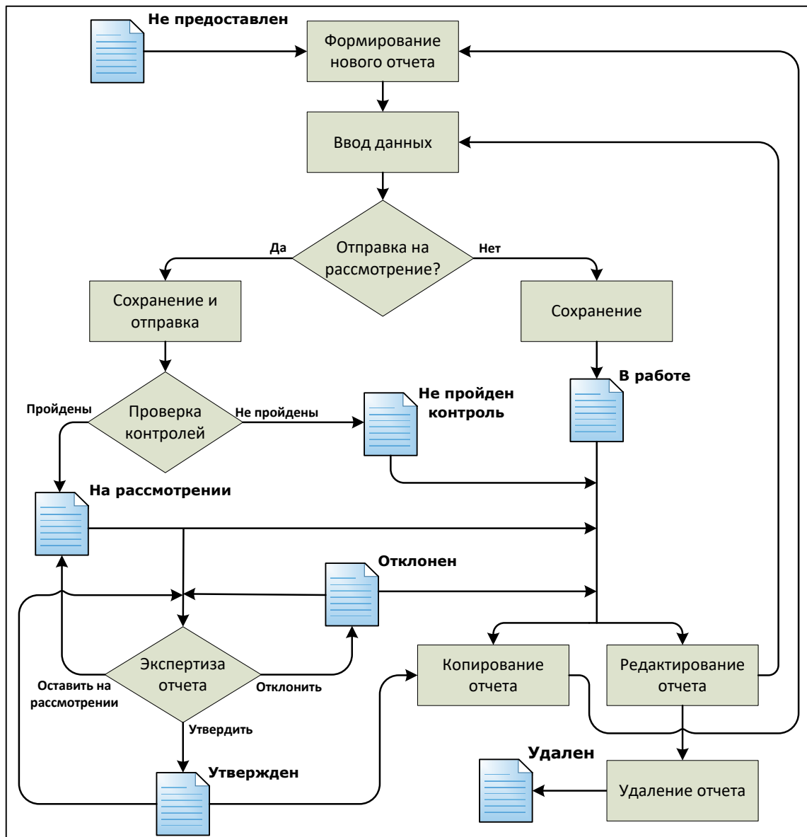
Рис. 1. Схема смены статусов отчета
